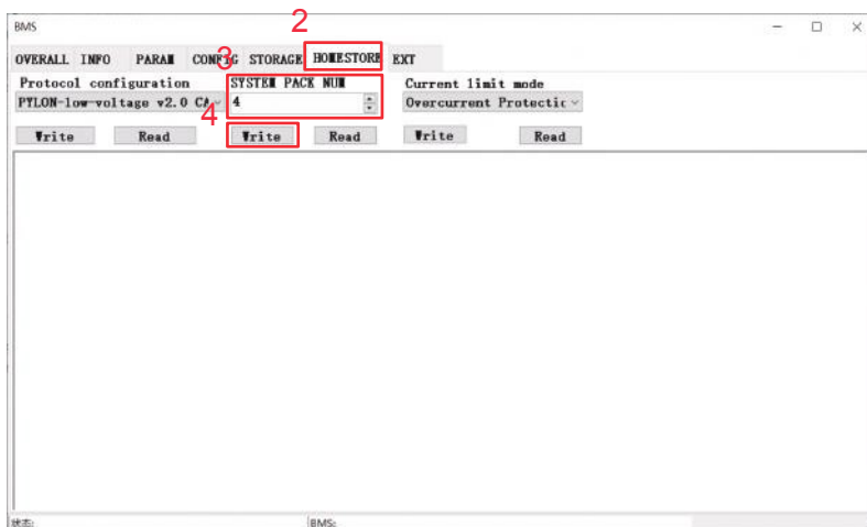
Figura 7-2 Pagina di configurazione
