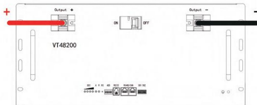
Figura 6-5 Collegamento del cavo di alimentazione del gruppo batteria
