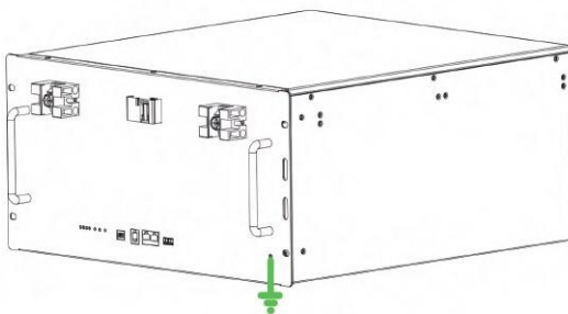
Figura 6-4 Collegamento del cavo di terra
