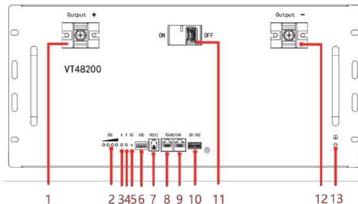
Figura 5-1 Pannello frontale
