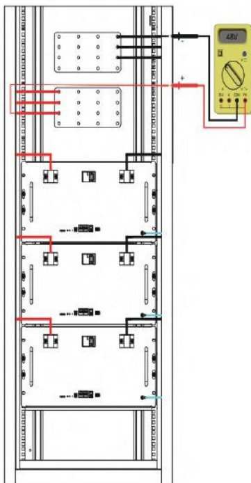
Figura 7-1 Controllo della tensione della batteria
