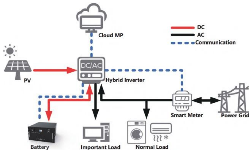
Figura 3-1 Schema di funzionamento normale del gruppo batteria
