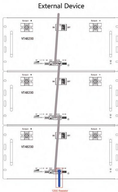
Figura 6-7 Collegamento della resistenza da 120Ω
